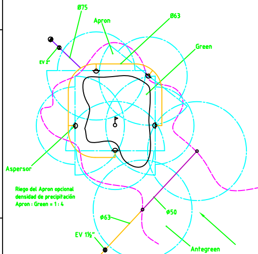
Distribución de Aspersores en el Green y Antegreen
