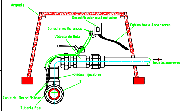
Esquema de instalación para el Green con aspersor de válvula incorporada
