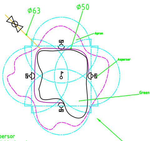
Distribución de Aspersores en el Green
