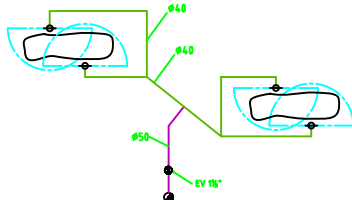
Distribución de Aspersores en el Tee
