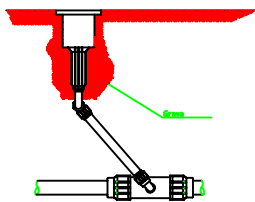
Conexión del Aspersor
