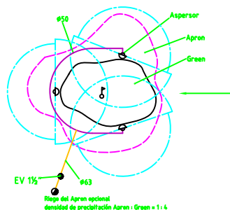
Distribución de Aspersores en el Green
